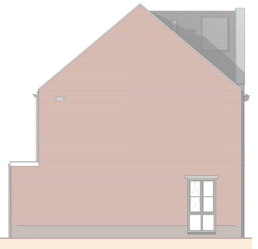
Linker zijgevel
